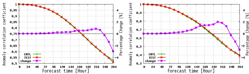
図4 北半球領域(北緯20度以北)における500hPa面ジオポテンシャル高度のアンサンブル平均予測のアノマリー相関係数とその改善率。左は冬実験、右は夏実験。赤線はTEST、緑線はCNTLのアノマリー相関係数、紫線はアノマリー相関係数の改善率(右縦軸)。横軸は予測時間(0~264時間)。
