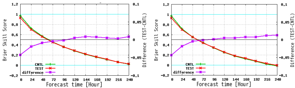
図6 図5に同じ。ただし赤線はLAF法を適用した54メンバー、緑線は適用しない27メンバーのブライアスキルスコア、紫線はスコアの差(右縦軸)。横軸は予報時間(0~240時間)。
