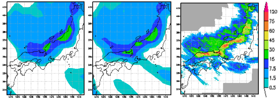
図3 平成23年12月26日12UTCを初期時刻とする72時間予測。ただし、前24時間降水量(単位:mm)。左からCNTL、TEST、対応する解析雨量。
