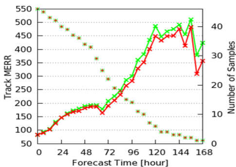
図2 夏実験における台風進路予報誤差(単位:km)の平均。赤線はTEST、緑線はCNTLの誤差、赤点は事例数、横軸は予報時間(0～168時間)。いずれも初期摂動を加えないコントロールメンバーの結果。
