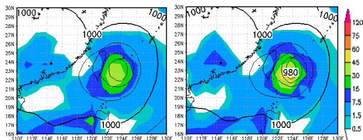
図1 台風の予測例。平成24年8月1日12UTCを初期時刻とする72時間予測(左: CNTL、右: TEST)。ただし、前6時間降水量(色、単位:mm)と海面気圧(4hPa毎等値線、単位:hPa)を表示。
