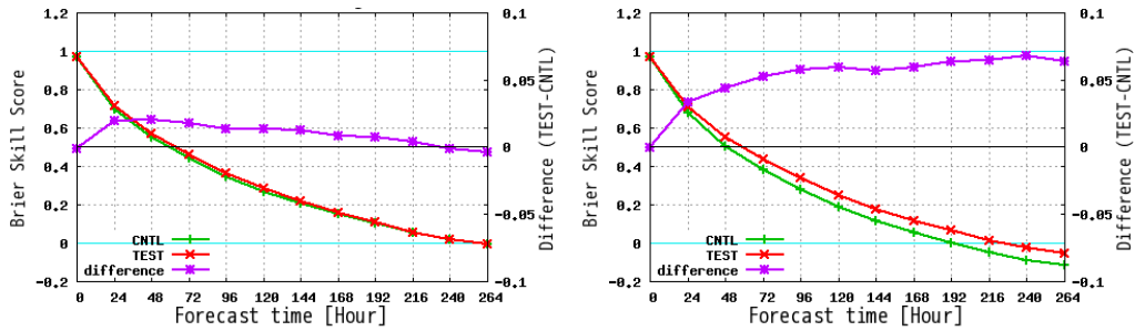
図5 夏実験の北半球領域(北緯20度以北)における850hPa面気温が高・低温偏差となる確率的予測のブライアスキルスコアとその差。左は高温偏差(偏差が \sigma (気候学的変動量)を上回る場合)予測、右は低温偏差(偏差が -\sigma を下回る場合)予測。赤線はTEST、緑線はCNTLのブライアスキルスコア、紫線はスコアの差(TEST-CNTL、右縦軸)。横軸は予報時間(0~264時間)。
